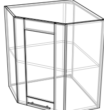
ШКАФ НАСТЕННЫЙ УГЛОВОЙ ВСТАВКА ЛДСП Д586xГ586xВ720
