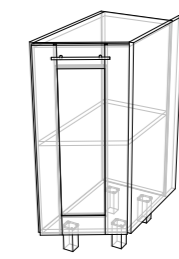
ПОСУДОМОЙКА НА 450 (ФАСАД) С ПЛАНКОЙ ВСТАВКА ЛДСП Д450xГ18xВ713
