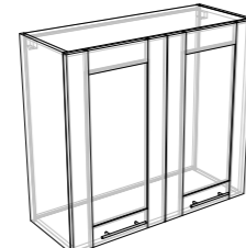
ШКАФ НАСТЕННЫЙ ПОД СУШКУ ВСТАВКА ЛДСП Д800xГ308xВ720
