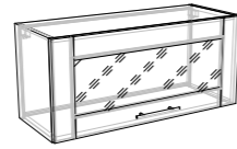
ШКАФ НАСТЕННЫЙ ГОРИЗОНТАЛЬНОЕ ОТКРЫВАНИЕ ВСТАВКА СТЕКЛО Д800xГ308xВ360
