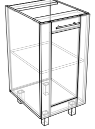
ПОСУДОМОЙКА НА 600 (ФАСАД) С ПЛАНКОЙ ВСТАВКА ЛДСП Д600xГ18xВ713
