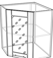
ШКАФ НАСТЕННЫЙ УГЛОВОЙ ВСТАВКА СТЕКЛО Д586xГ586xВ720
