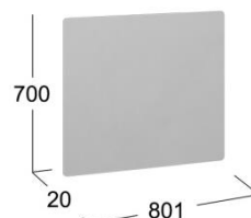
Панель с зеркалом ТД – 297.06.02
