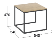
Стол журнальный тип 2 Бунратти/Черный
