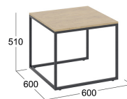
Стол журнальный тип 1 Бунратти/Черный
