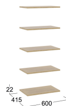
Комплект полок 600 Бунратти
