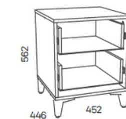
HM 041.11 Прикроватная тумба
