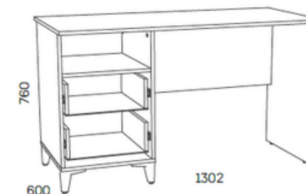
HM 041.16 Стол письменный (возможна право- и левосторонняя сборка)
