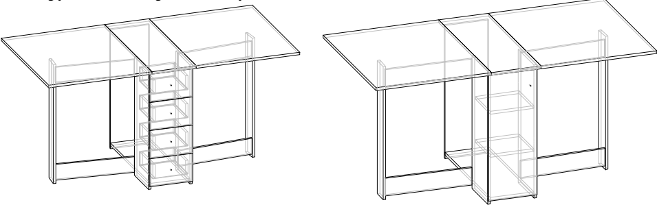
ШхВхГ 340(1700)х780х880 рис.1.
