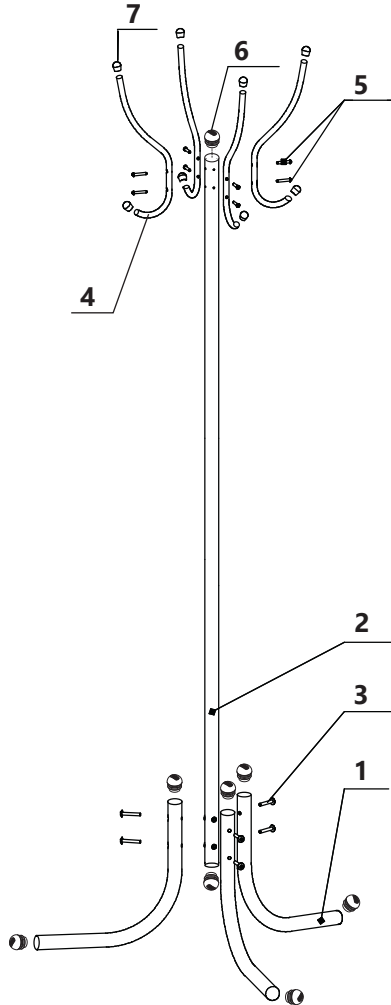
Рис. 1 Схема сборки
